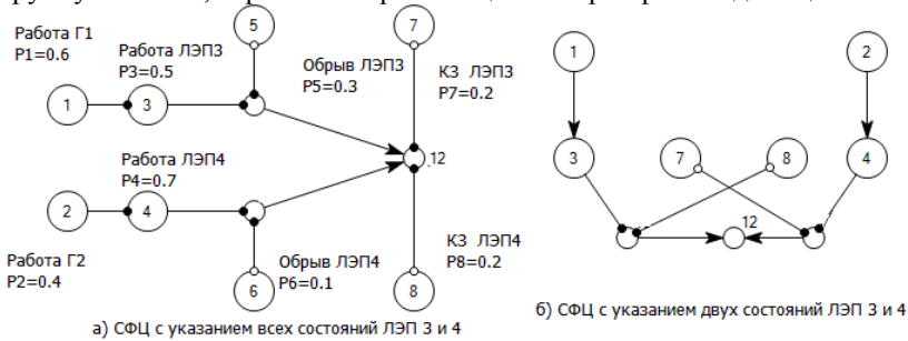
Рис.5. СФЦ энергетической системы [3].
